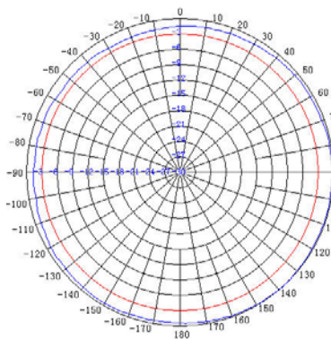
Horizontal Beamwidth
