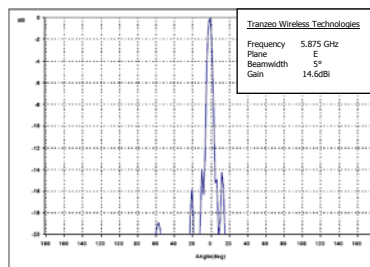
E-Plane
