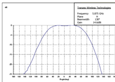
H-Plane
