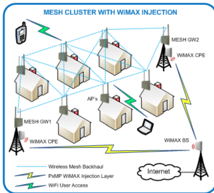
网状网和wimax混合组网示意图
